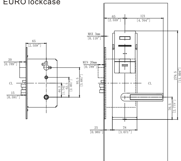
EURO lockcase
