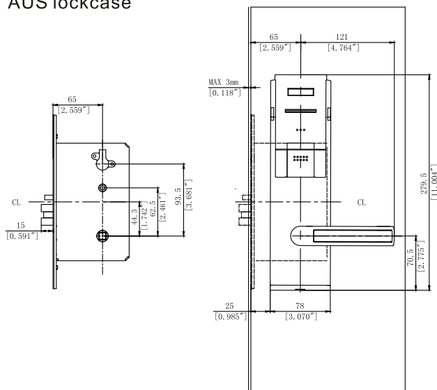
AUS lockcase
